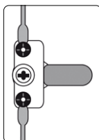
7 Fermeture 3 points : elle est composée d'une serrure à came multipoints et d'un système à tringles. En verrouillant la fermeture, elle actionne les 3 points de condamnation de la porte (haut, milieu et bas), offrant ainsi une sécurité maximale.
