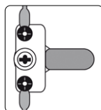
7 Fermeture 3 points : elle est composée d'une serrure à came multipoints et d'un système à tringles. En verrouillant la fermeture, elle actionne les 3 points de condamnation de la porte (haut, milieu et bas), offrant ainsi une sécurité maximale.
